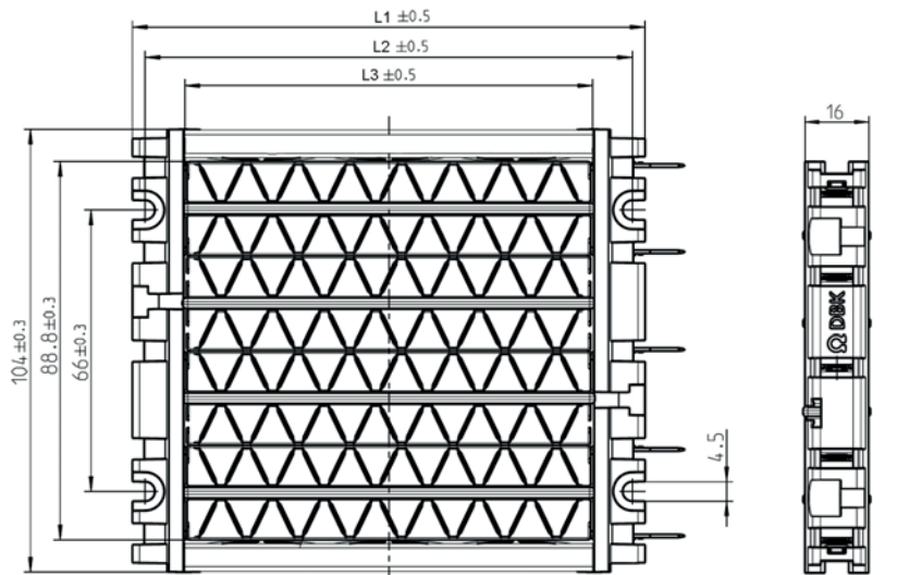
Vorderansicht neues Gehäuse
